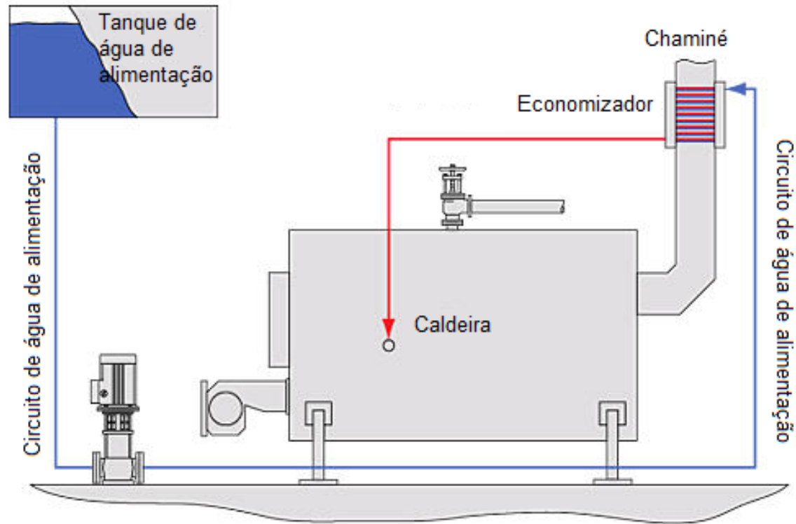
Figura 27.6 Economizador de uma caldeira flamotubular
