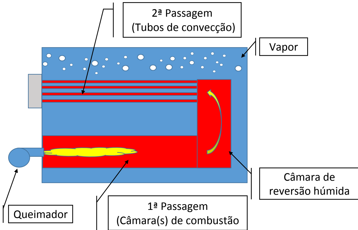
Figura 27.4 Caldeira com câmara de reversão húmida
