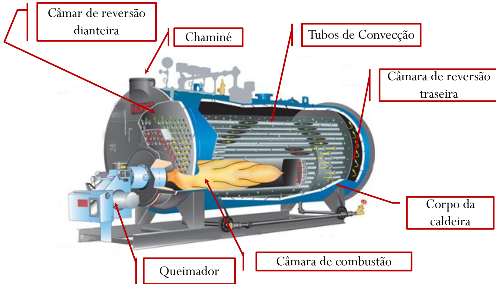
Figura 27.1 Partes principais da caldeira flamotubular
