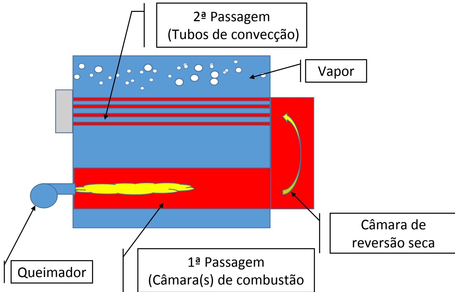
Figura 27.3 Caldeira com câmara de reversão seca
