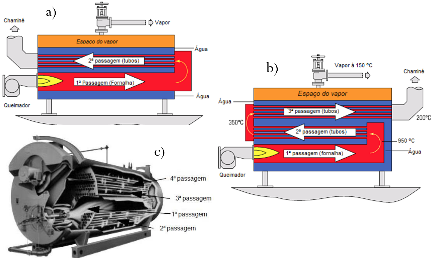
Figura 27.2 Caldeiras com duas a), três b) e quatro c) passagens
