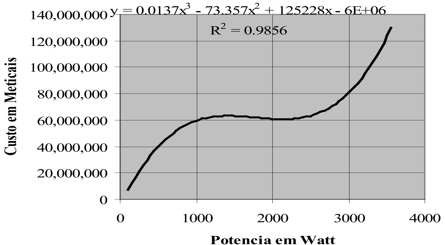
Grafico 1. Custos em função da potência
