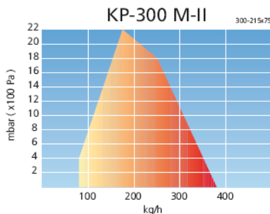
Figura 18.26 Gráficos de capacidade/contrapressão para queimadores à combustível líquido
