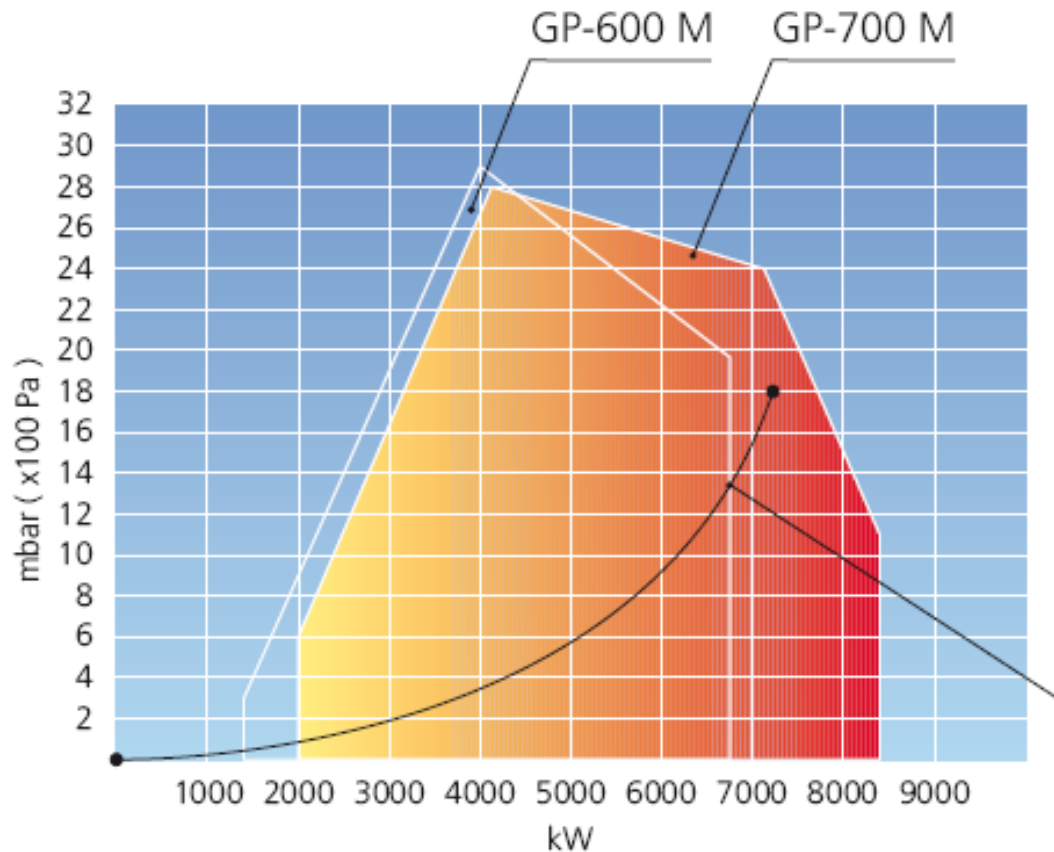
Gráfico de perda de pressão da caldeira em função da capacidade do queimador
