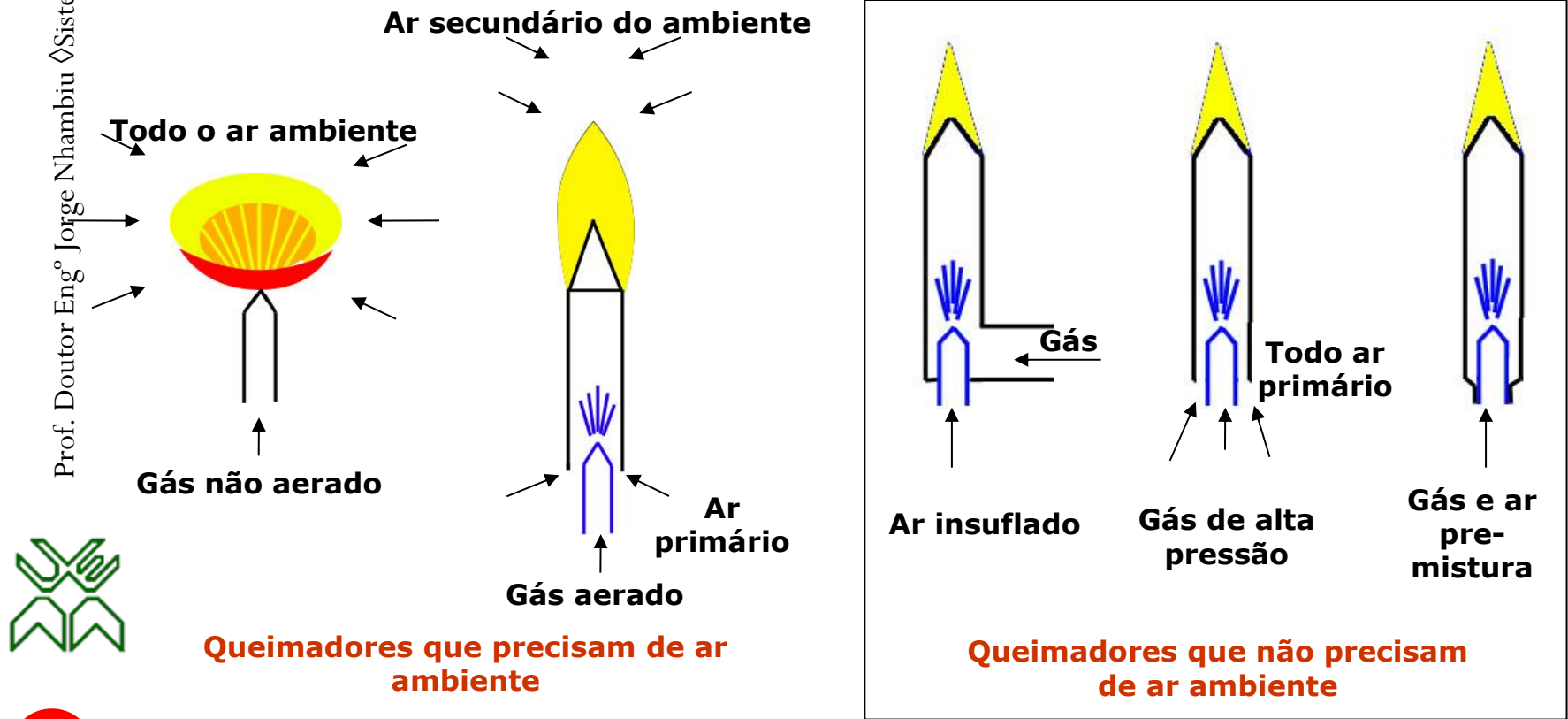
Figura 18.2 Exemplo de queimadores
