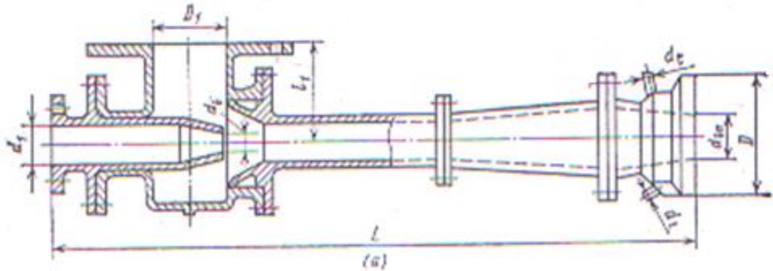
Figura 18.6 Queimadores com pré-aquecimento
