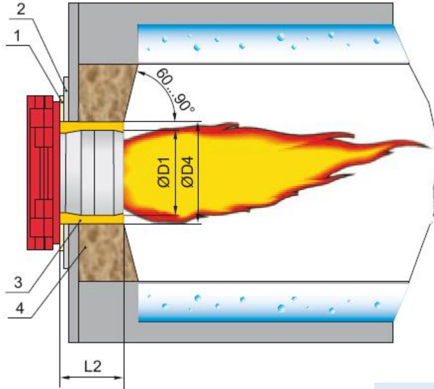
Figura 18.23 Corte transversal em figura da alvenaria
