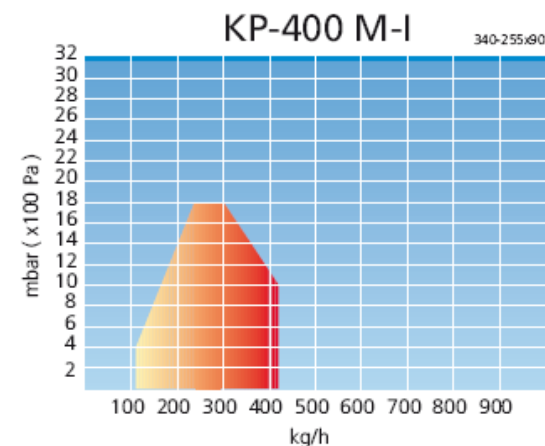
Figura 18.26 Gráficos de capacidade/contrapressão para queimadores à combustível líquido
