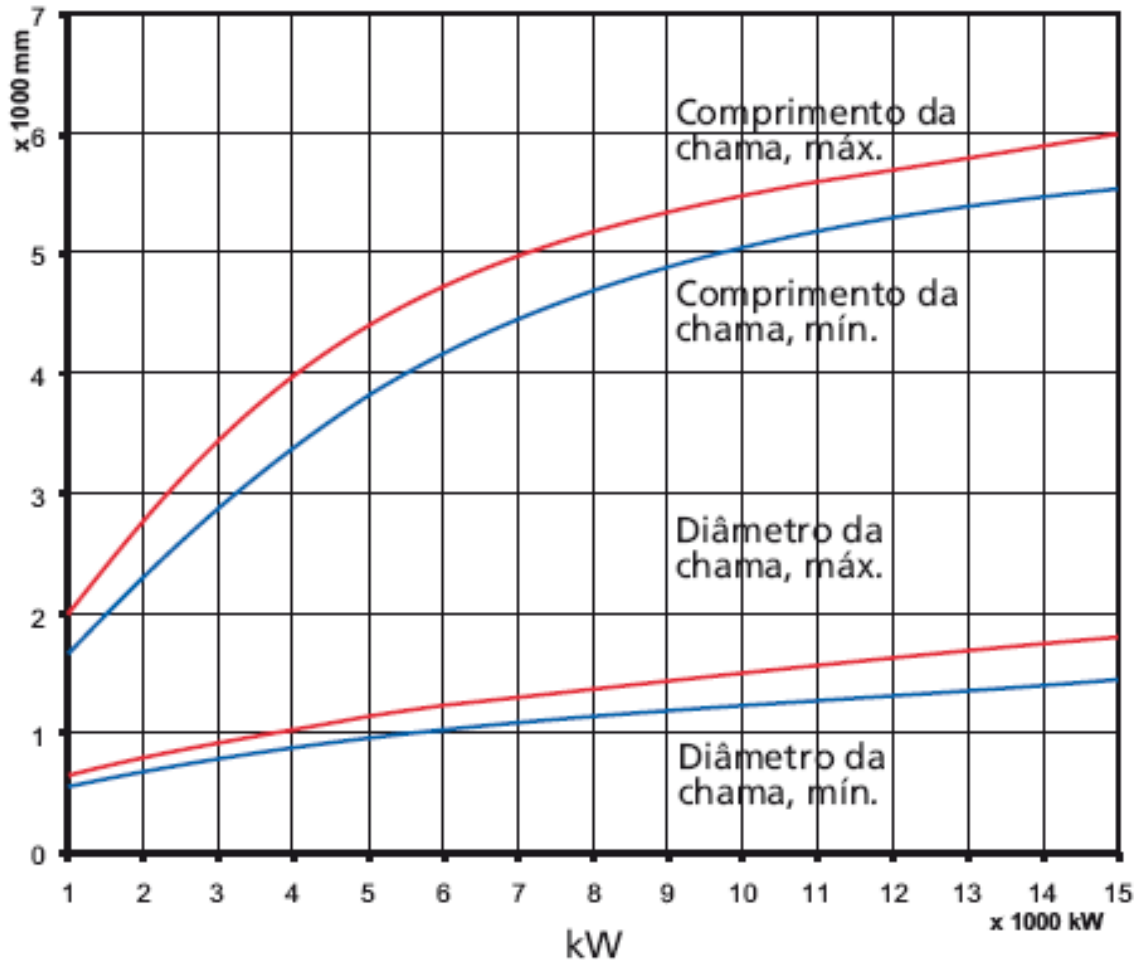
Figura 18.24 Características da chama em função da potência do queimador
