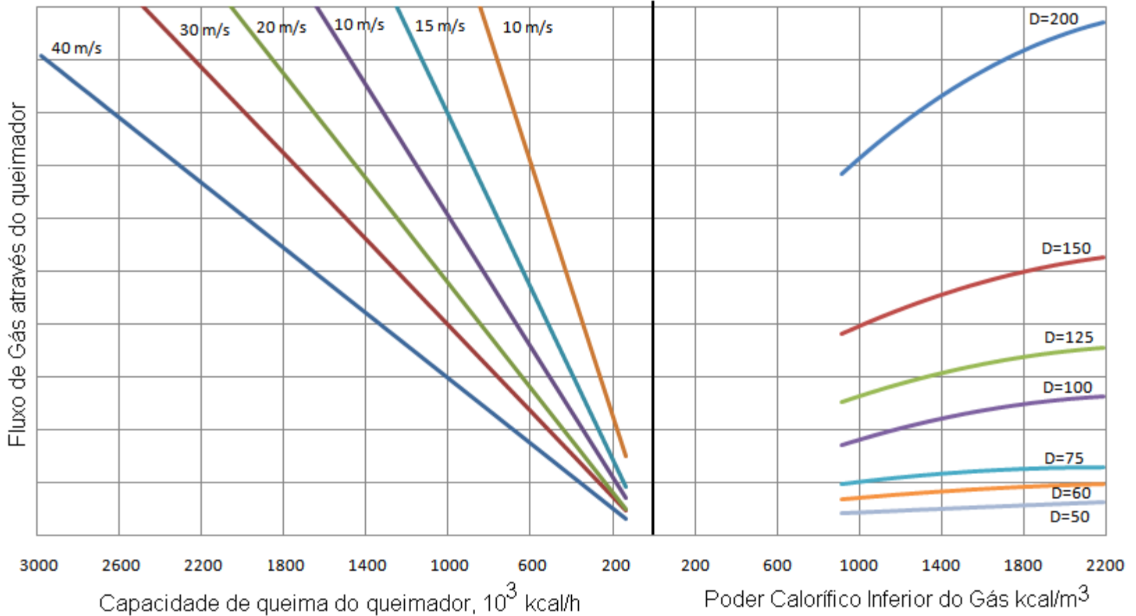
Figura 18.12 Monograma para seleccionar queimadores turbulentos
