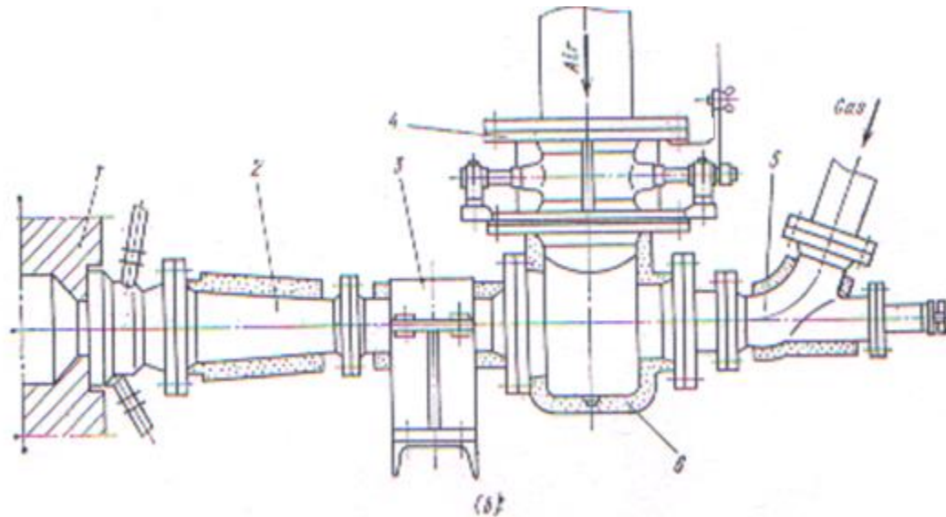
Figura 18.8 Queimadores com pré-aquecimento
