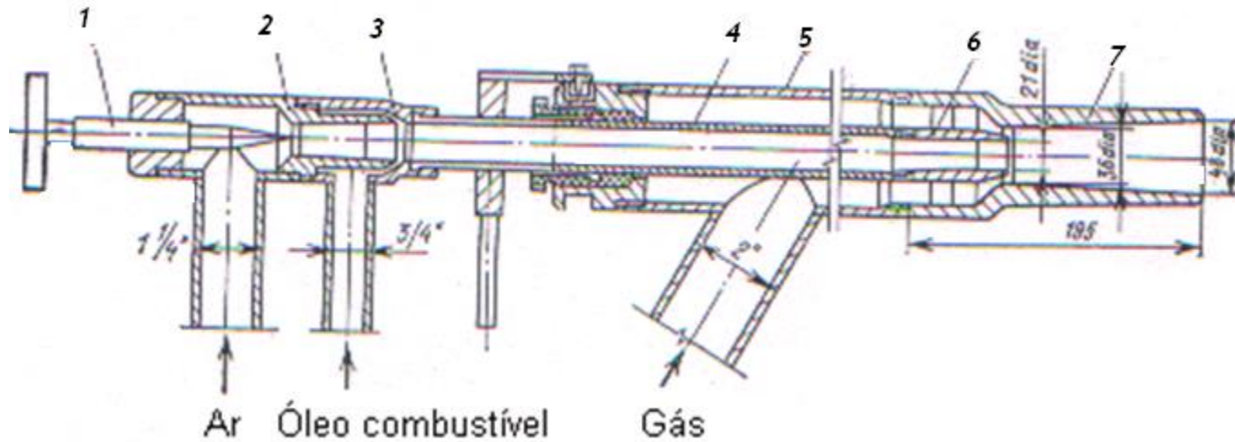
Figura 18.19 Queimador misto gás-líquido
