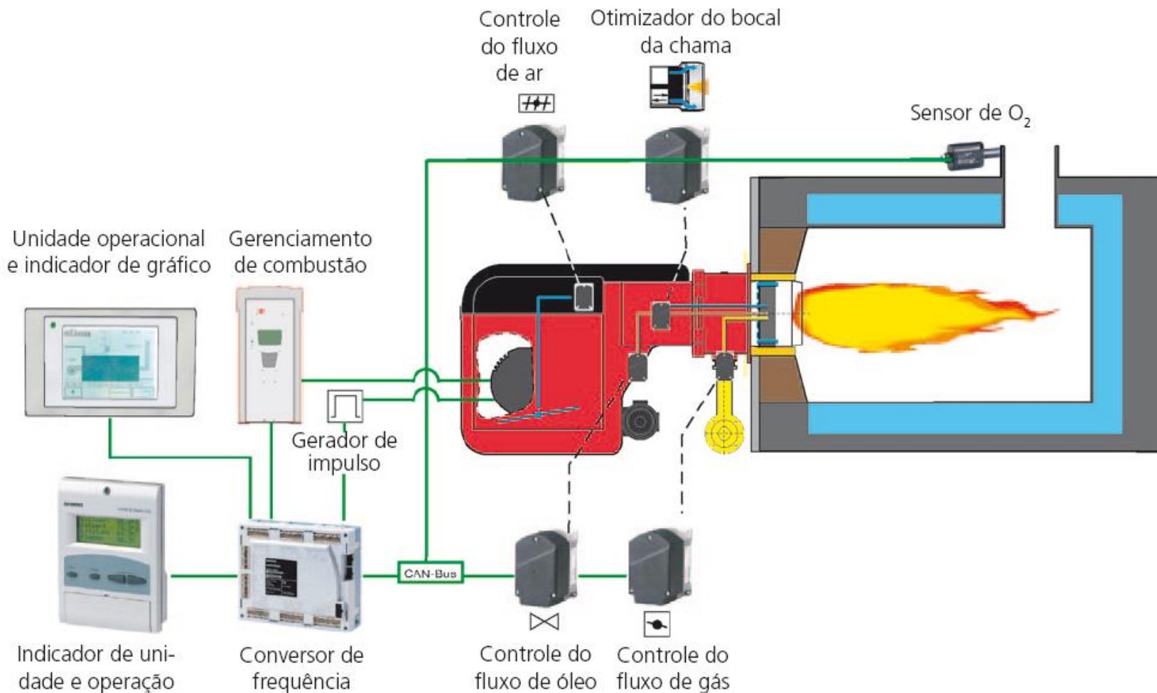
Figura 18.22 esquema geral de uma instalação de queimador
