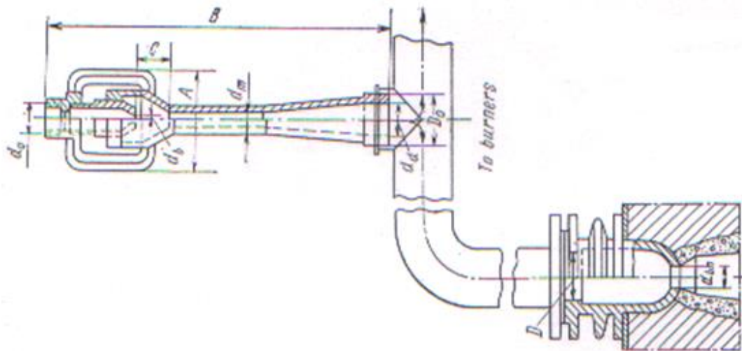
Figura 18.4 Misturador para vários queimadores
