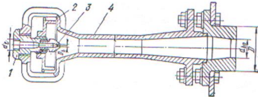
Figura 18.5 Queimador com misturador incorporado
