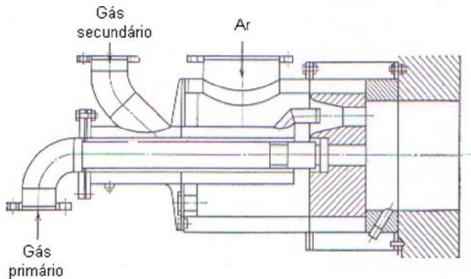
Figura 18.14 Queimadores com controle de comprimento da chama
