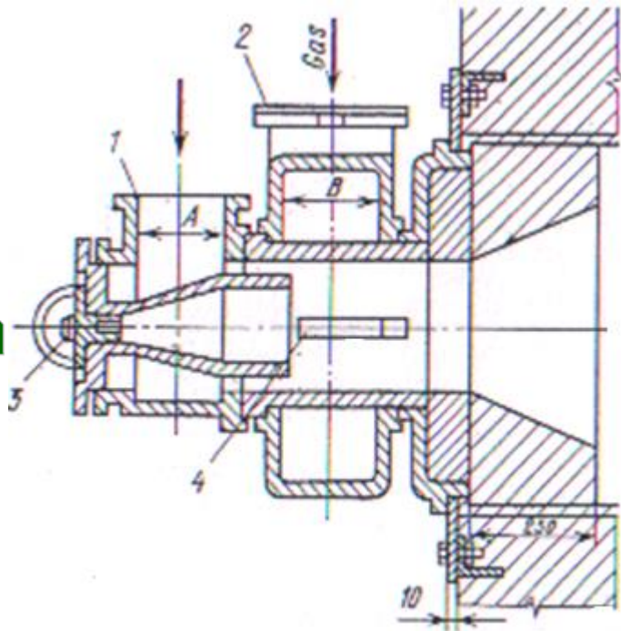
Figura 18.9 Queimador com mistura parcial
