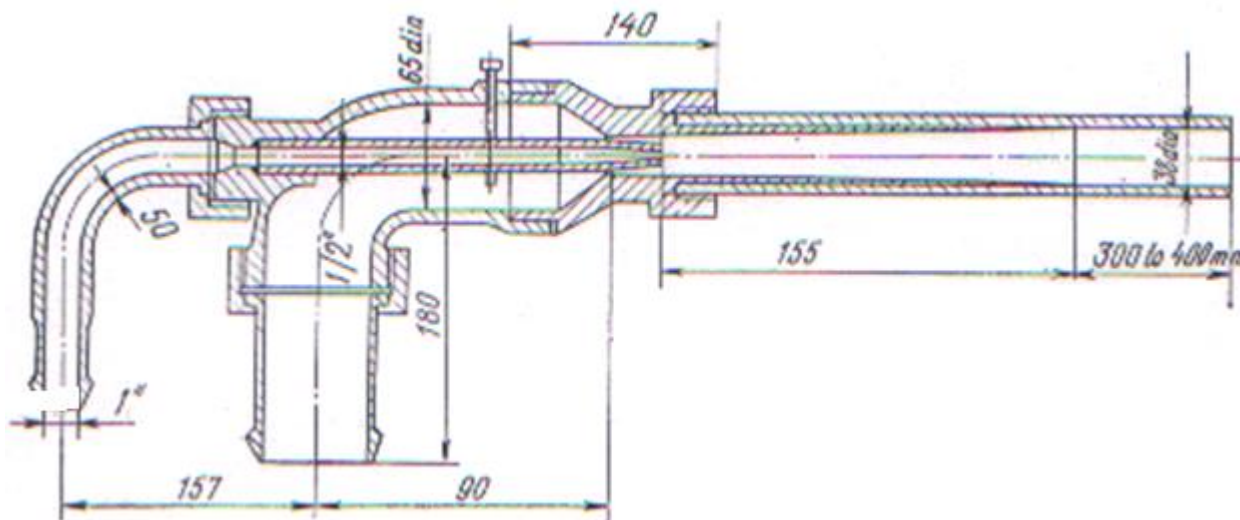
Figura 18.18 Queimador de alta pressão
