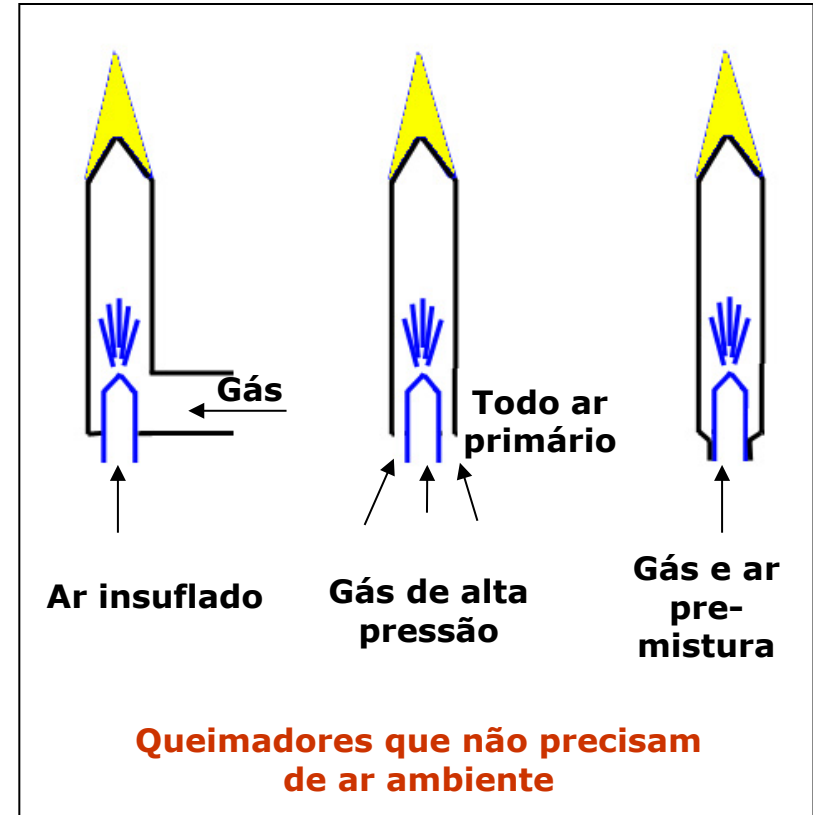
Figura 16.2 Exemplo de queimadores
