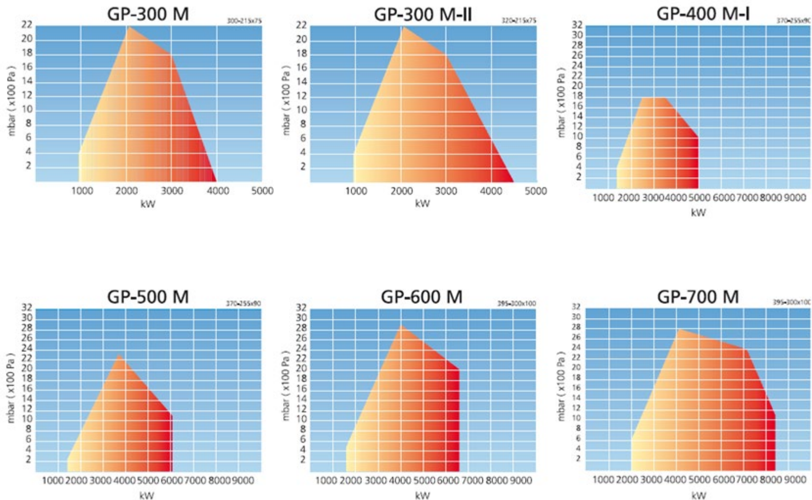
Figura 16.25 Gráficos de capacidade/contrapressão para queimadores à gás
