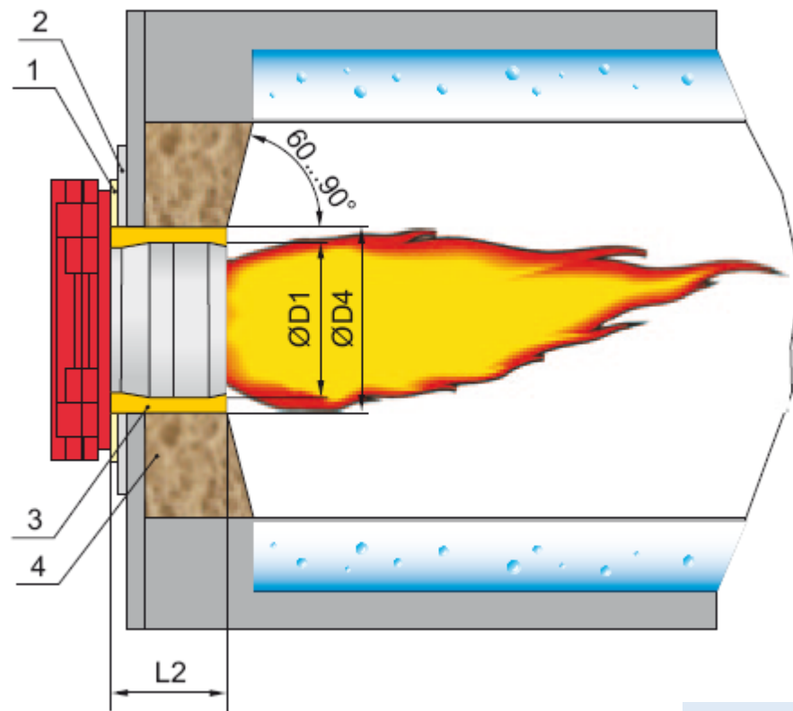
Figura 16.23 Corte transversal em figura da alvenaria
