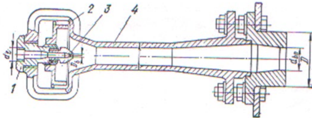
Figura 16.5 Queimador com misturador incorporado
