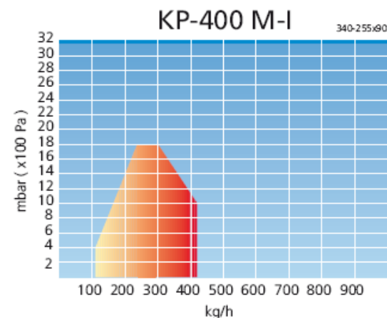
Figura 16.26 Gráficos de capacidade/contrapressão para queimadores à combustível líquido
