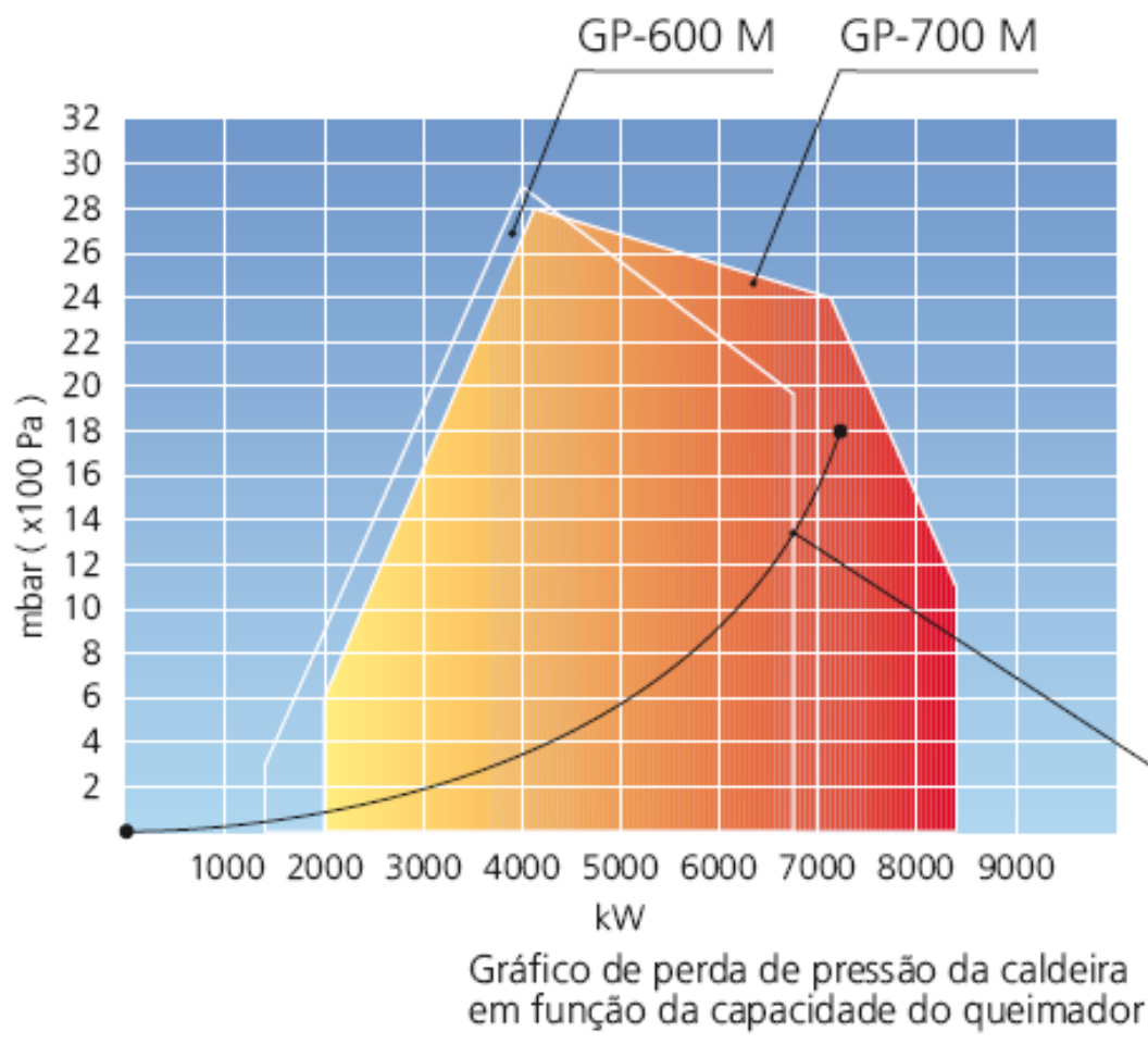
Figura 16.21 Gráfico de capacidade versus contrapressão
