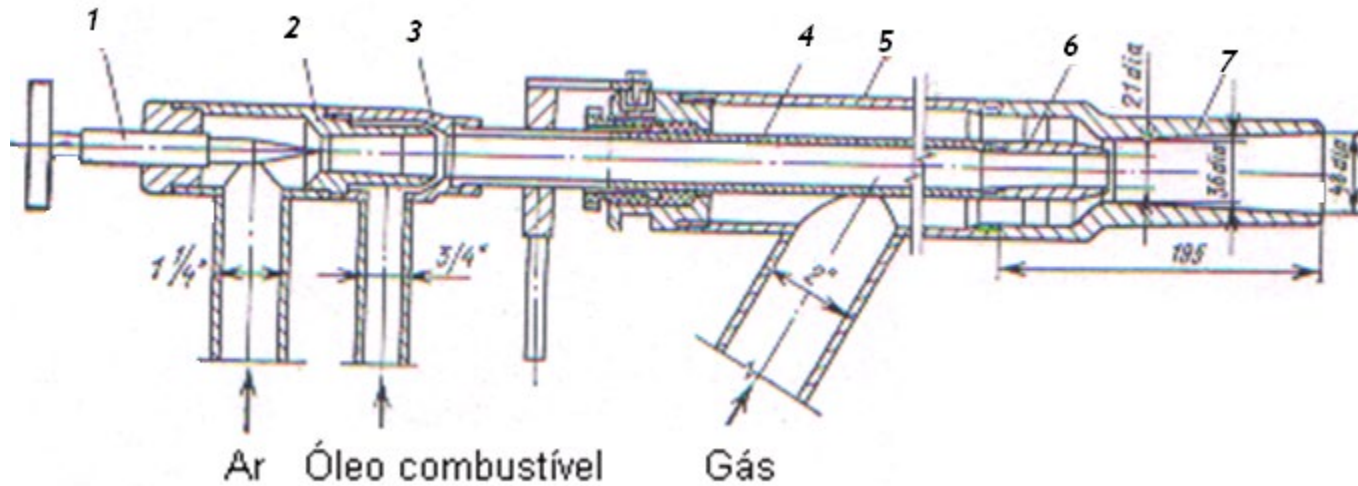
Figura 16.19 Queimador misto gás-líquido
