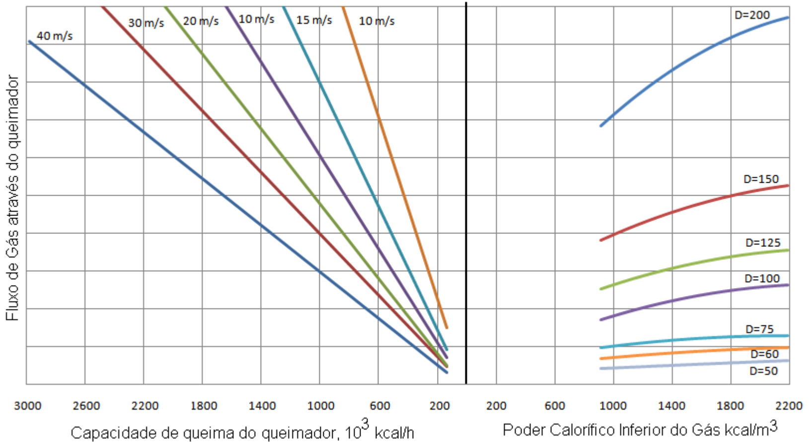
Figura 16.12 Monograma para seleccionar queimadores turbulentos
