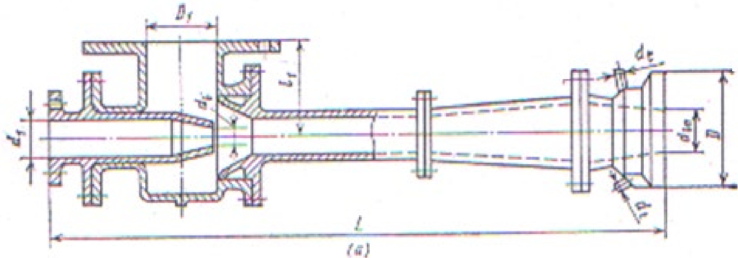
Figura 16.6 Queimadores com pré-aquecimento
