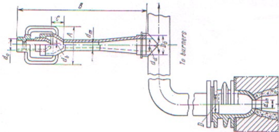
Figura 16.4 Misturador para vários queimadores
