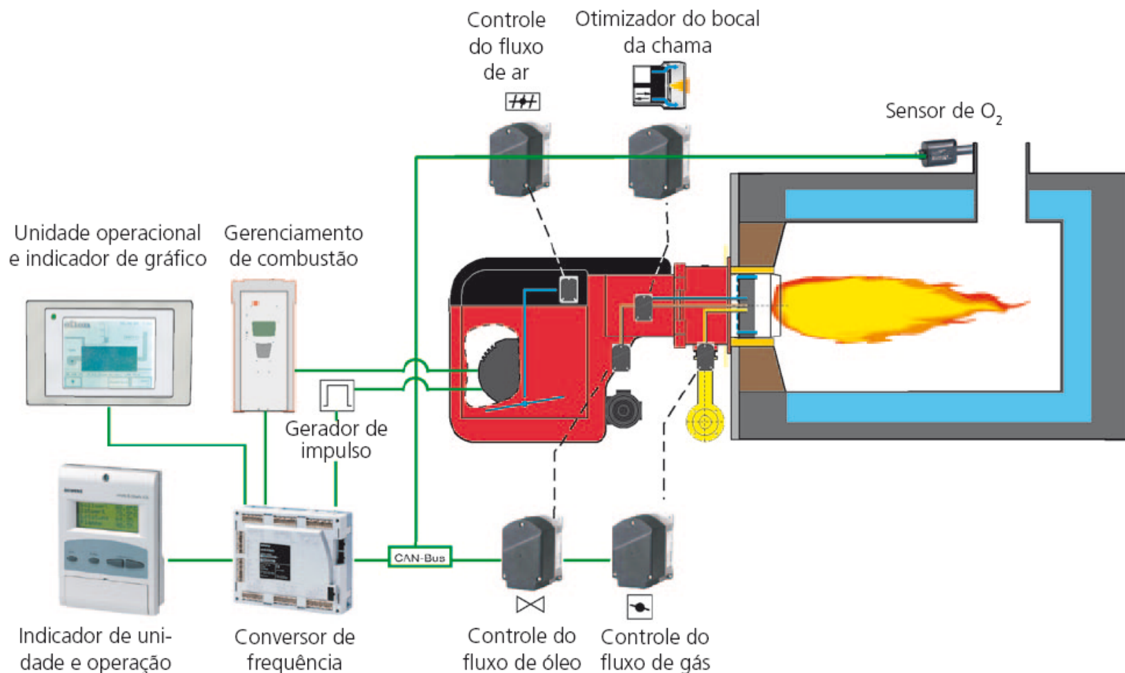
Figura 16.22 esquema geral de uma instalação de queimador
