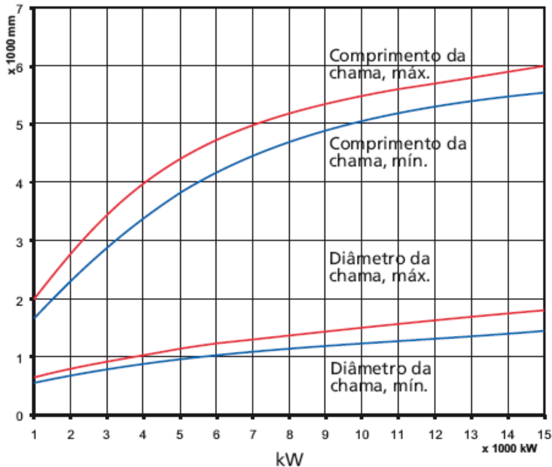
Figura 16.24 Características da chama em função da potência do queimador
