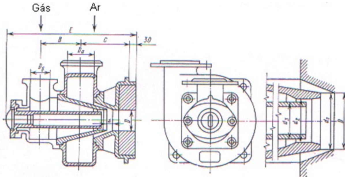
Figura 16.11 Queimador Turbulento
