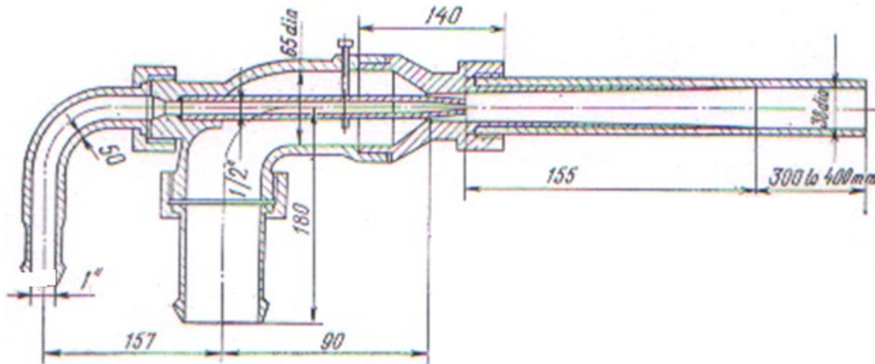
Figura 16.18 Queimador de alta pressão
