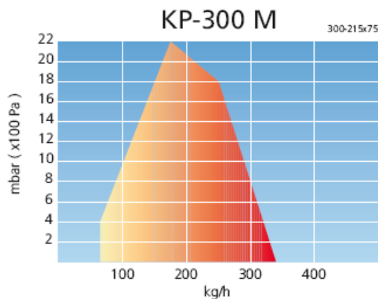
Figura 16.26 Gráficos de capacidade/contrapressão para queimadores à combustível líquido
