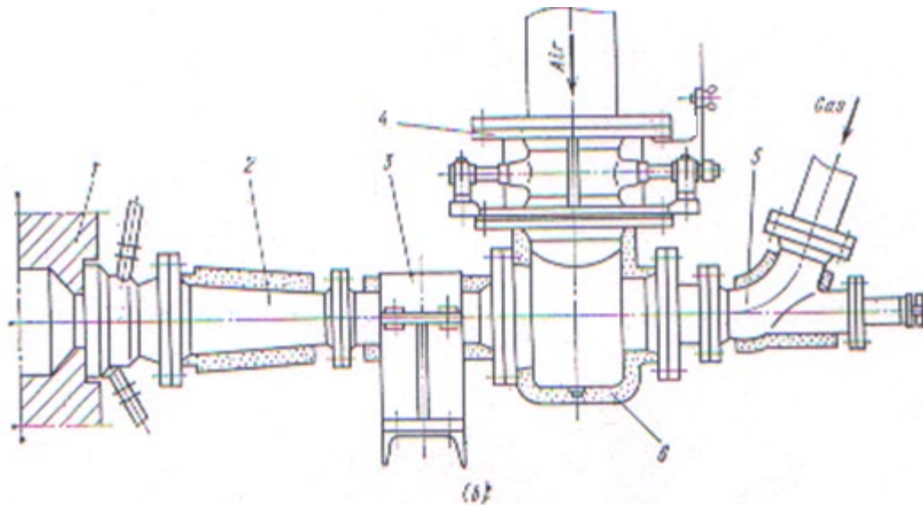
Figura 16.8 Queimadores com pré-aquecimento
