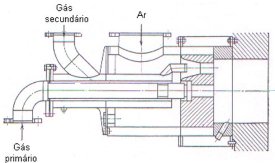
Figura 16.14 Queimadores com controle de comprimento da chama
