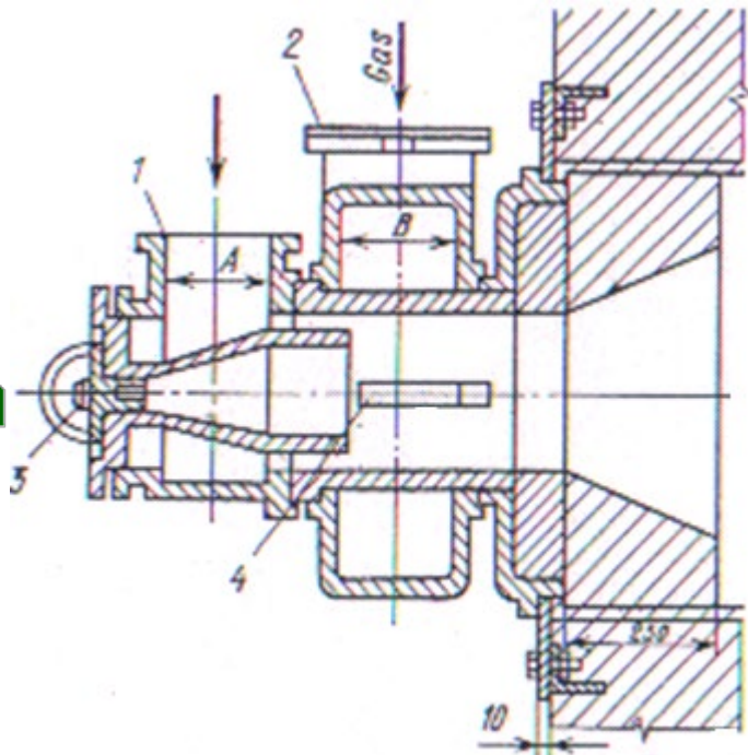
Figura 16.9 Queimador com mistura parcial
