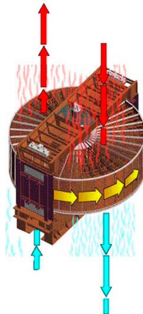
Figura 11.26 Aquecedor de ar Regenerativo
