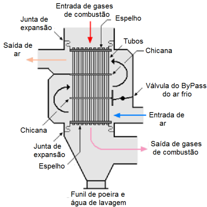
Figura 11.25 Aquecedor de ar Recuperativo
