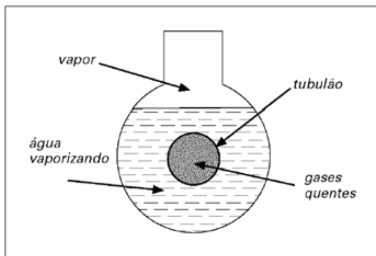
Figura 11.7 Caldeiras de tubos horizontais
