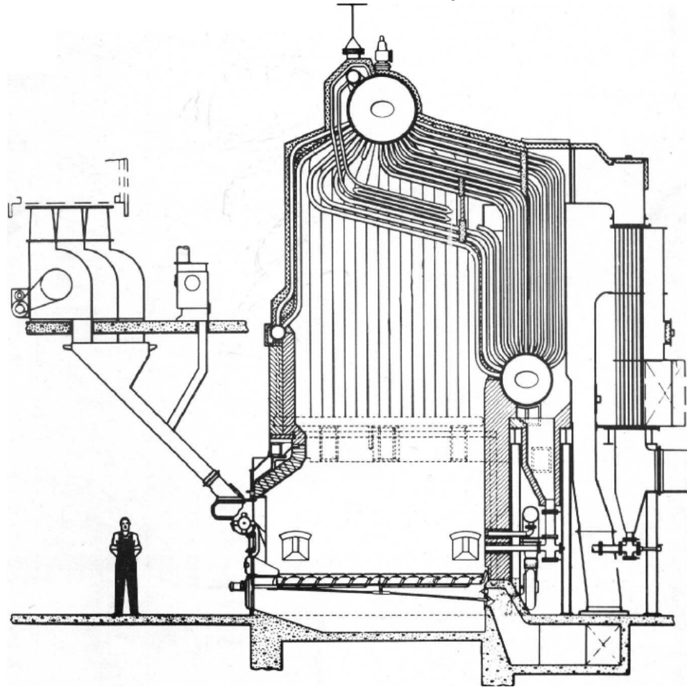
Figura 11.14 Caldeira Aquatubular em corte
