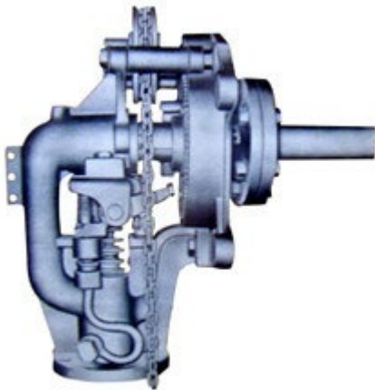
Figura 11.30 Sopradores de Fuligem
