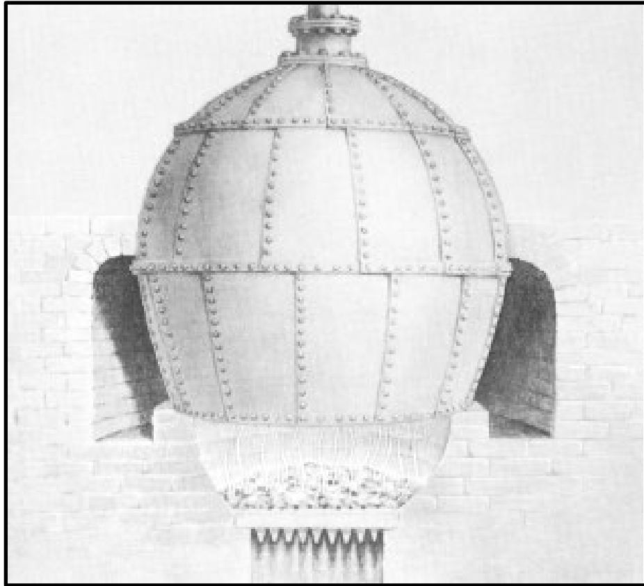
Figura 11.4 Caldeira de Haycock, 1720
