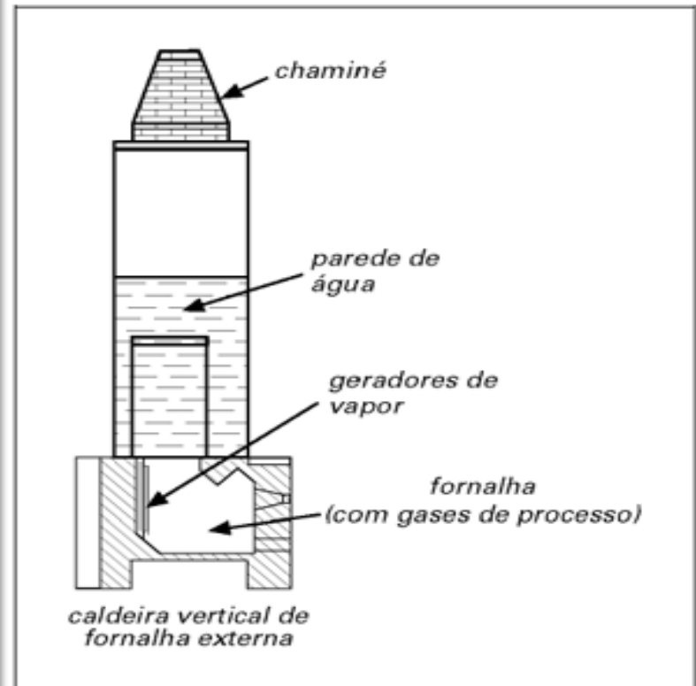
Figura 11.5 caldeira de tubos verticais
