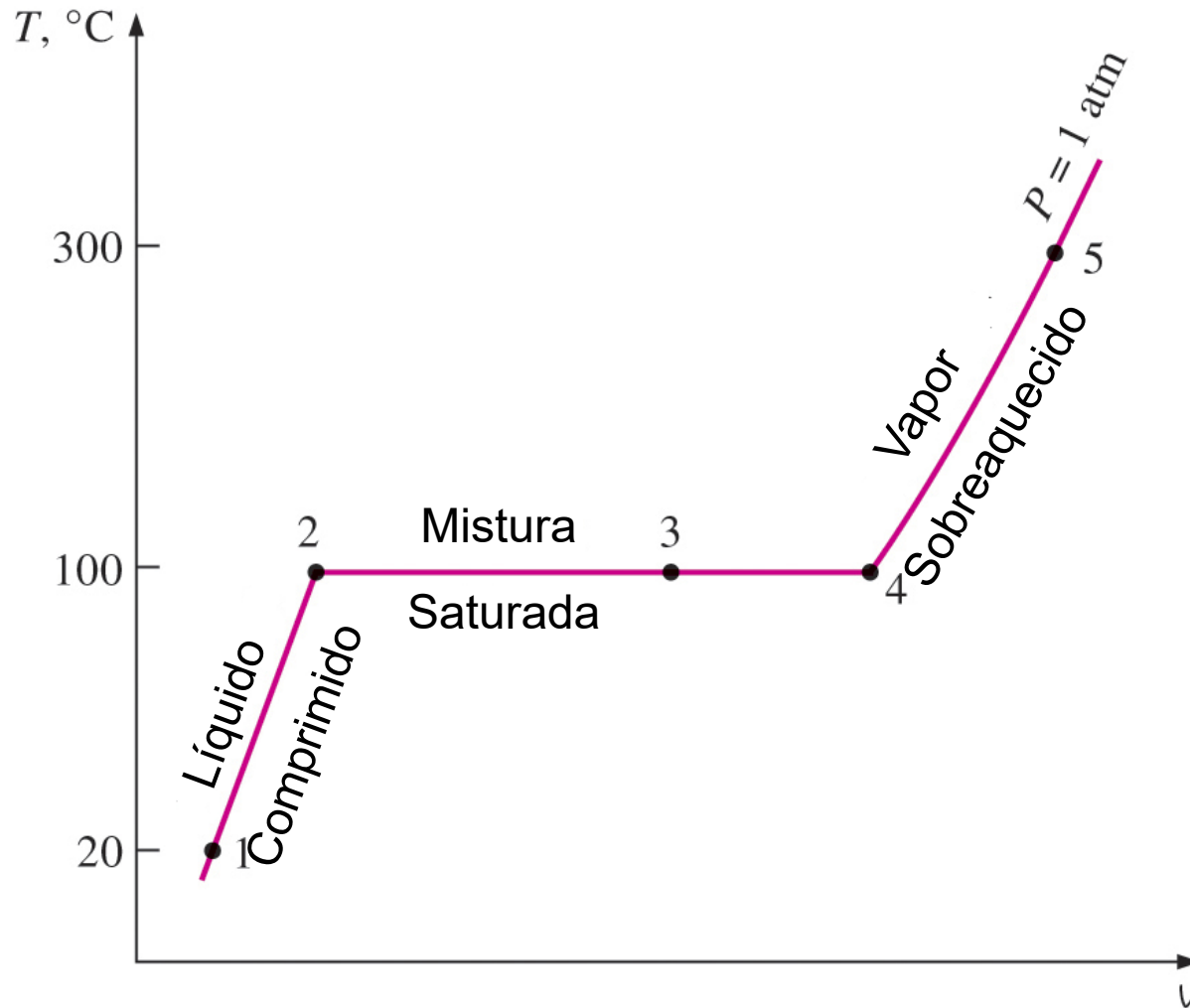
Figura 11.2 Diagrama T-v do processo
