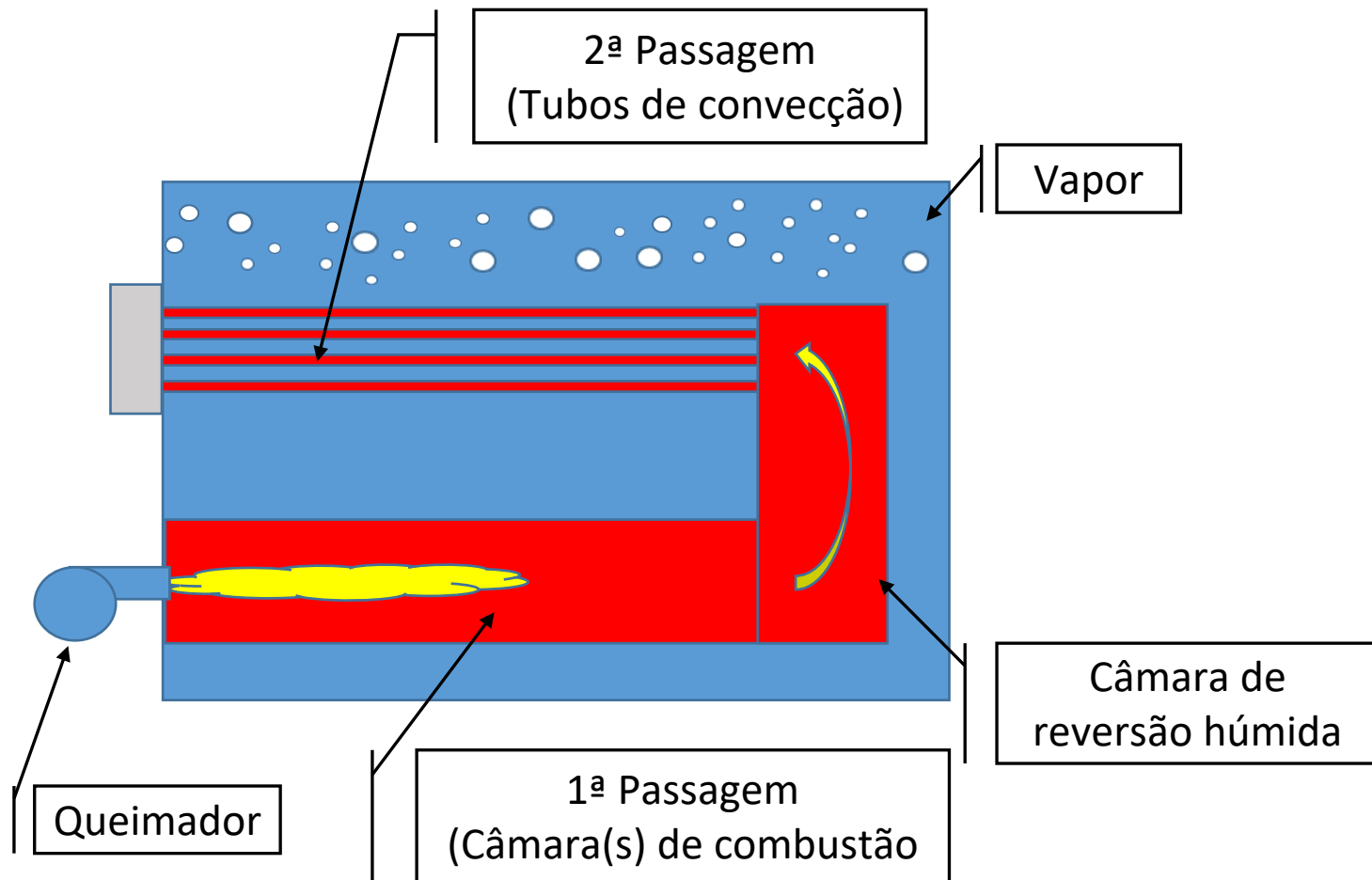
Figura 11.12 Caldeira com câmara de reversão húmida
