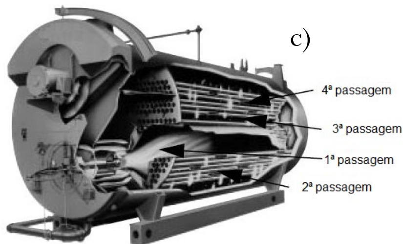
Figura 11.10 Caldeiras com duas a), três b) e quatro c) passagens
