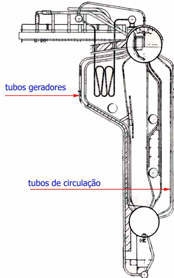
Figura 11.18 Circuitos da água nas Paredes de água
