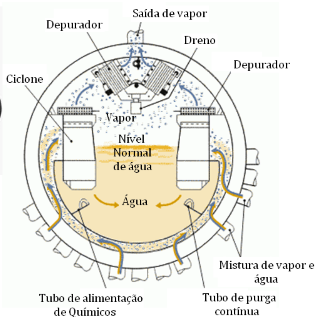
Figura 11.19 Tubulão superior
