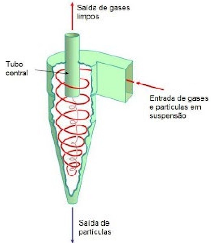
Figura 11.20 Ciclone
