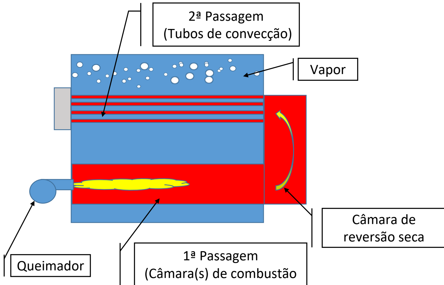
Figura 11.11 Caldeira com câmara de reversão seca
