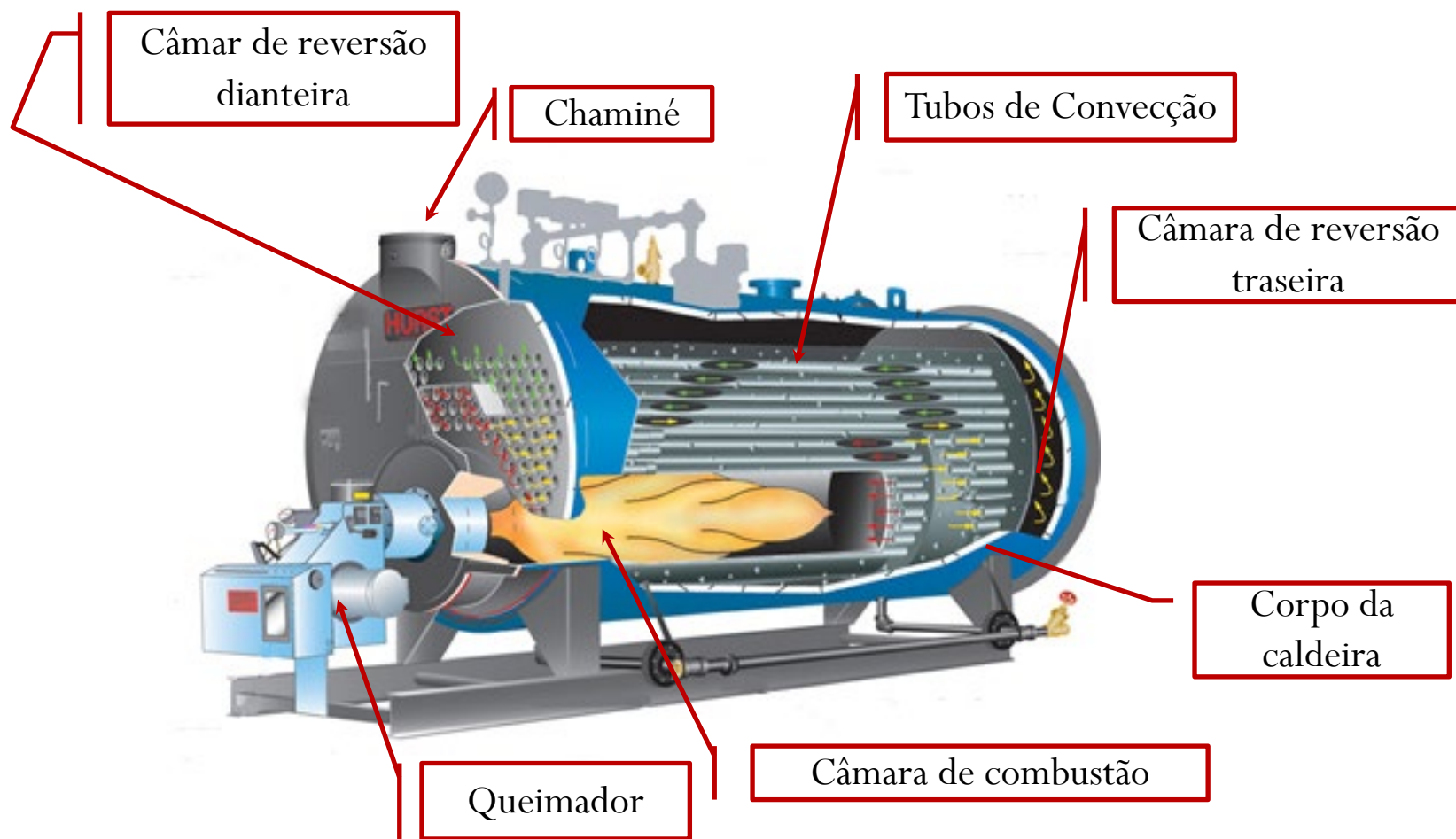
Figura 11.9 Partes principais da caldeira flamotubular
