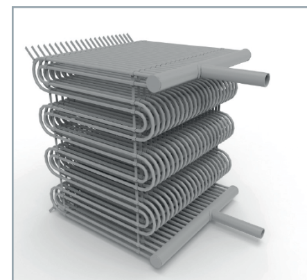
Figura 11.22 Superaquecedor Convectivo
